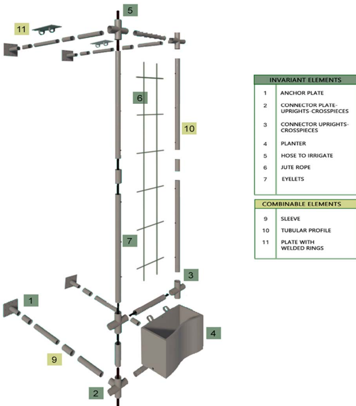
Fig. 1 – Esploso assometrico del prototipo
