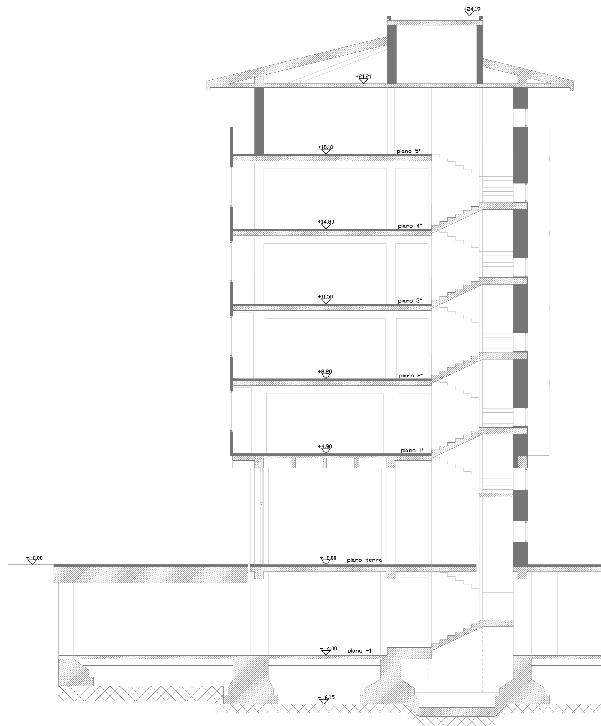
Sezione trasversale E-O
